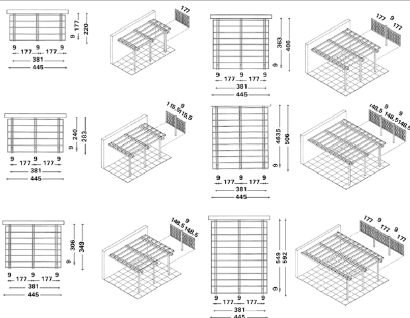
pergola L 445
