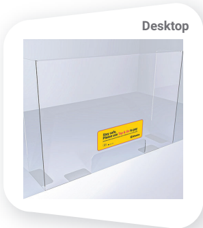
Covid Sneeze Screen 700mm (w) x 550mm (h) x 150mm (d)
